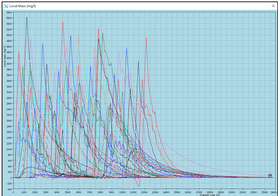
图 5.3.4-4 双茶亭、圆墩背稀土矿区矿块开采硫酸根离子浓度随时间变化曲线
