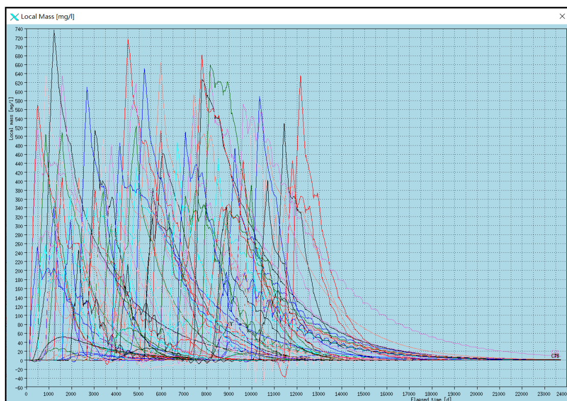
图 5.3.4-2 双茶亭、圆墩背稀土矿区矿块开采镁离子浓度随时间变化曲线图
