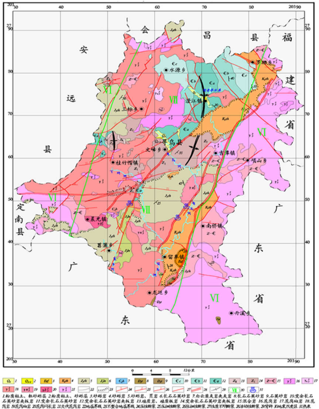
图 2.4.1-1 地质构造
