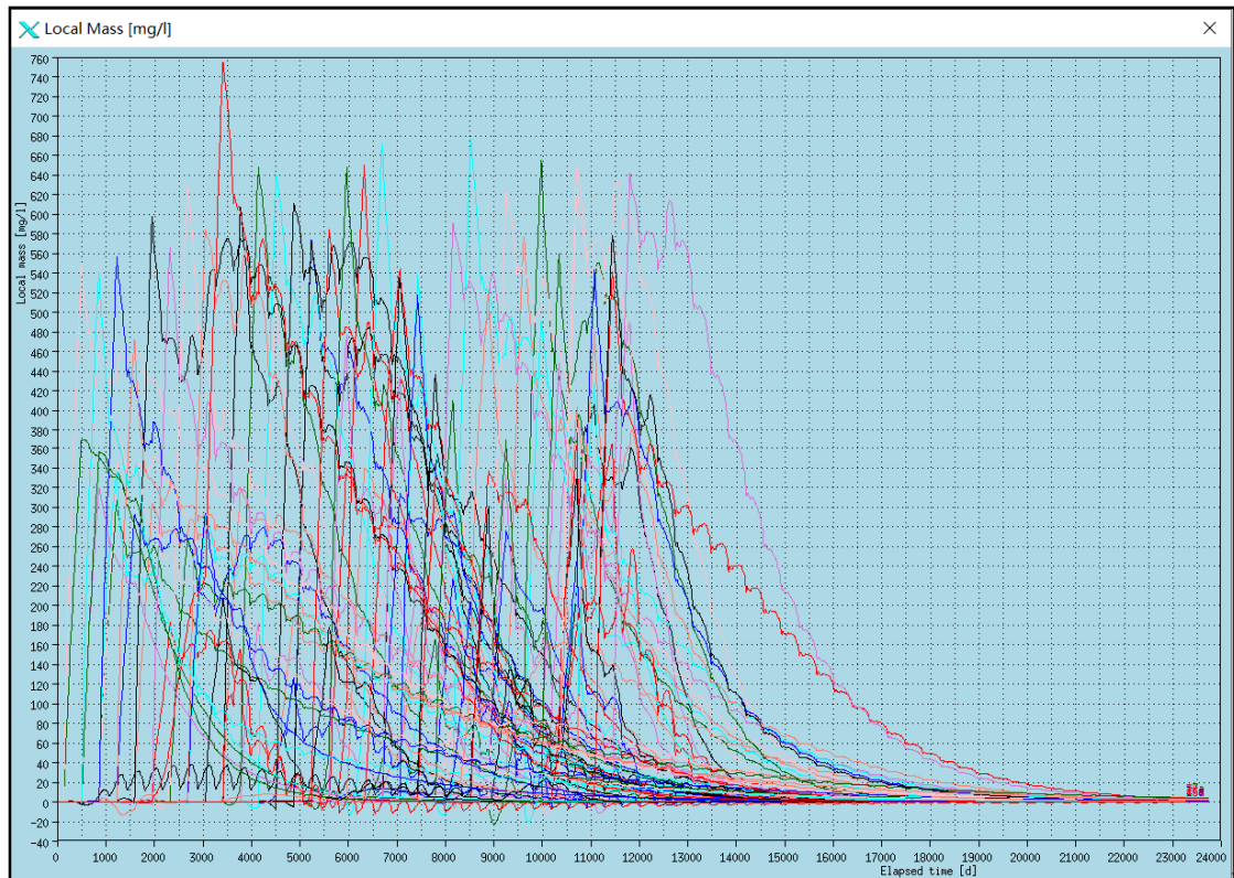
图 5.2.4-2 柯树塘矿区矿块开采镁离子浓度随时间变化曲线图
