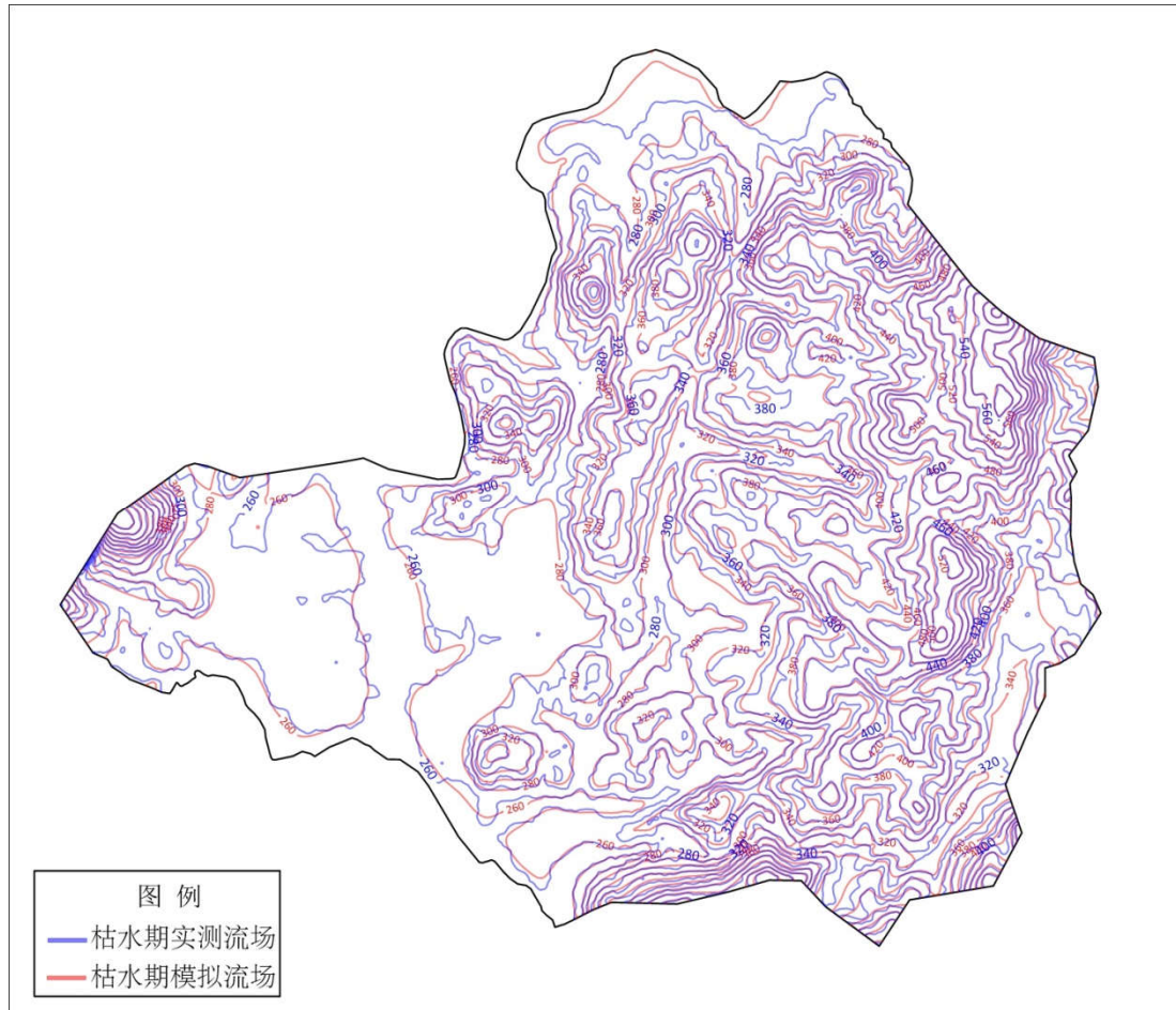
图 5.3.2-6 模拟区枯水期实测等水位线与计算等水位线对比图 (2021.11)
