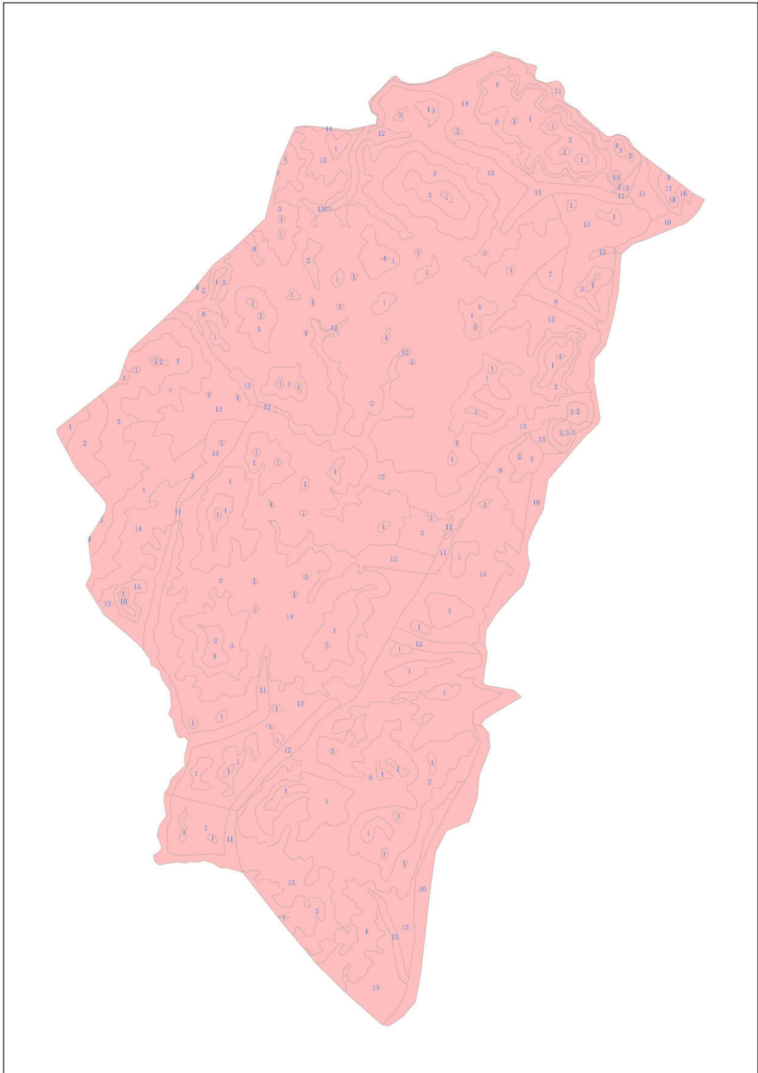
图 5.2.2-4 柯树塘模拟区含水层渗透系数分区
