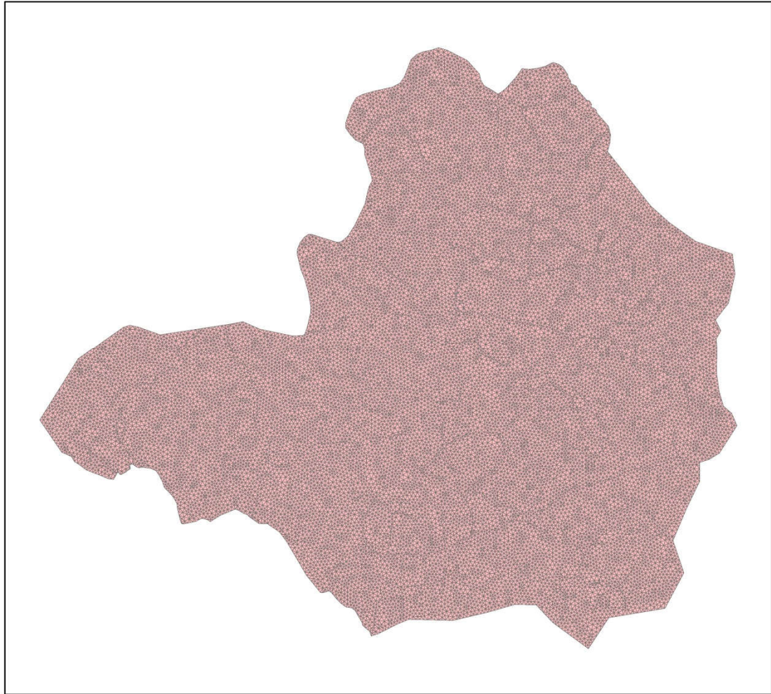
图 5.3.2-1 模型网格剖分图
