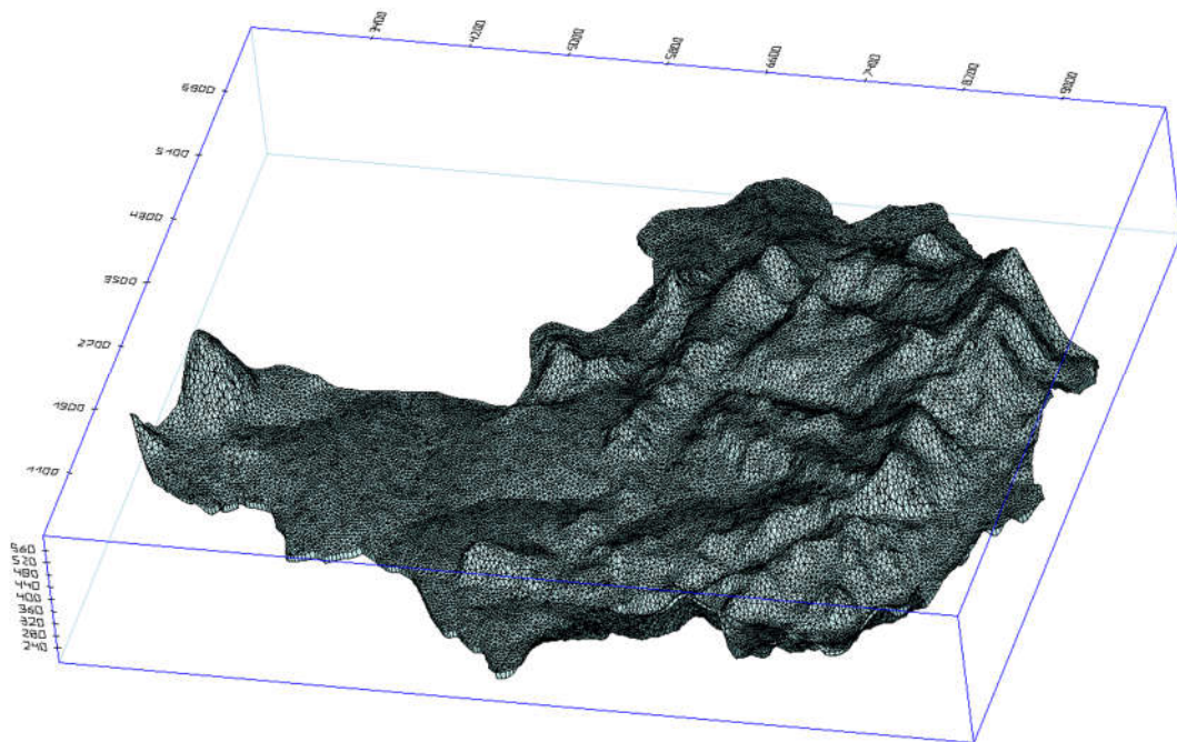
图 5.3.2-2 地下水渗流模型的网格剖分立体图 (2) 降雨入渗系数分区
